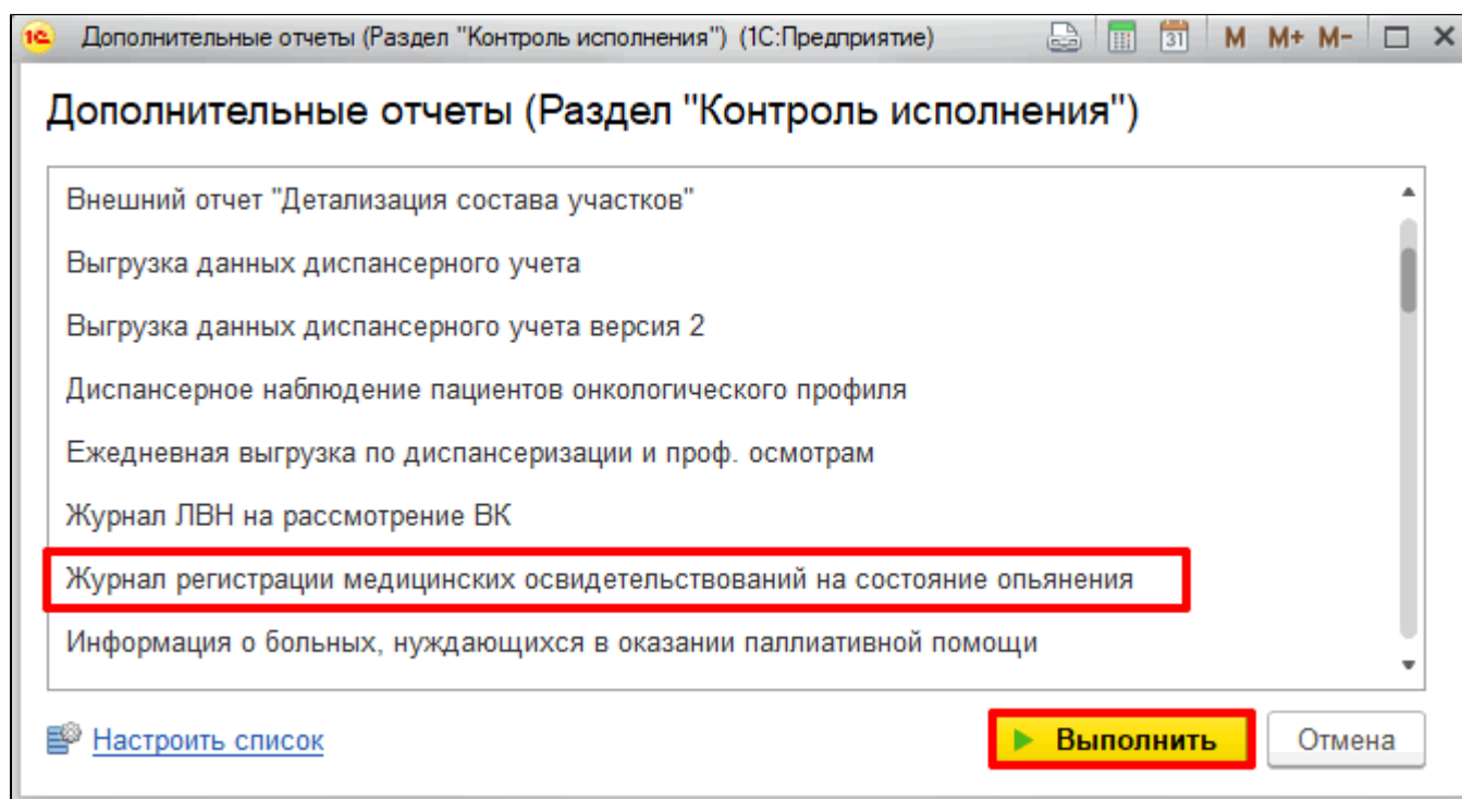
Рисунок 2. Дополнительные отчеты
