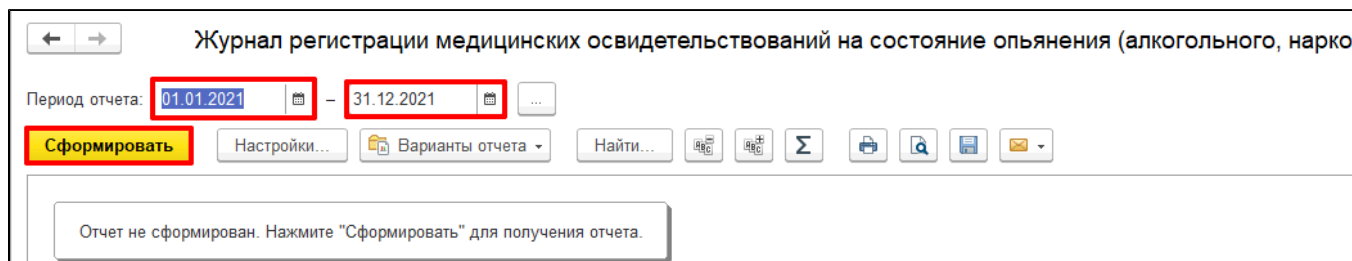
Рисунок 3. Формирование отчета
