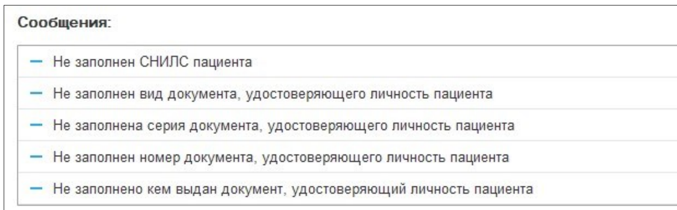
Рис. 3 – Предупреждающие сообщения
