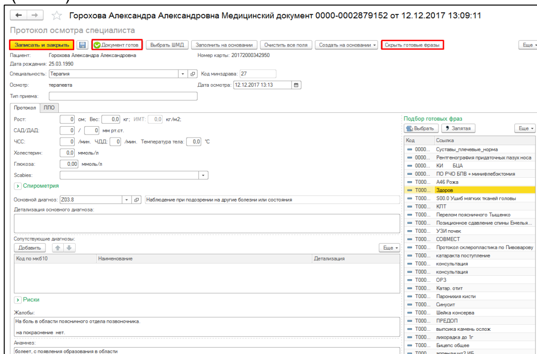
Рис. 4 – Заполнение документа
