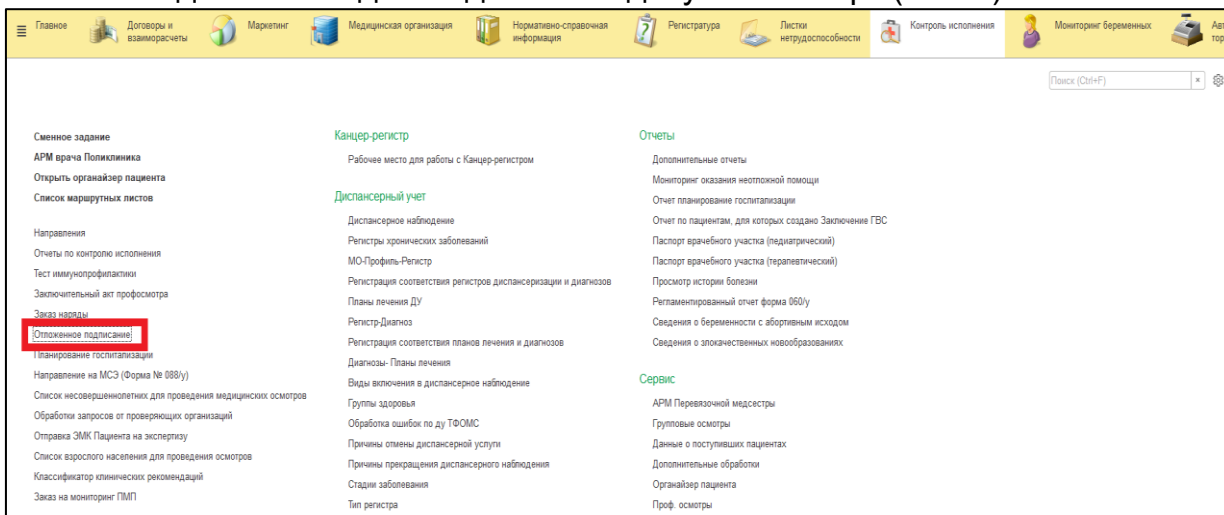
Рис. 7 – Отложенное подписание
